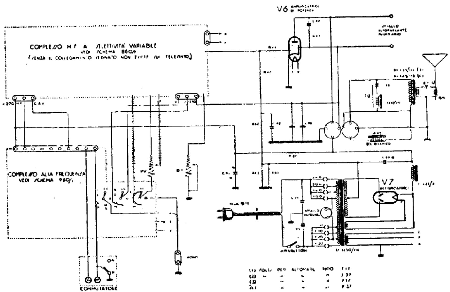
PHONOLA (S. A. FIMI) — Mod. "960" — Particolari dell'amplificatore a bassa frequenza.
